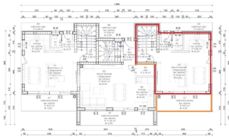
TLOCRT PRIZEMLJA mjerilo 1:500
